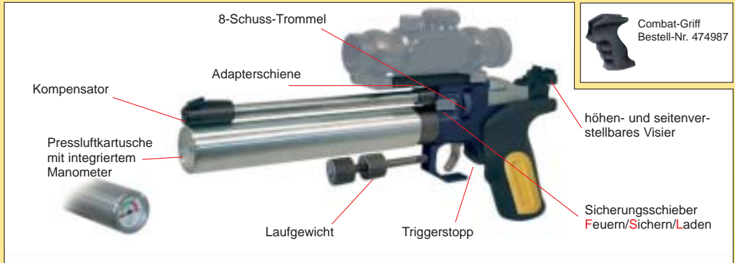
Pressluft-Set Bestell-Nr. 234949
